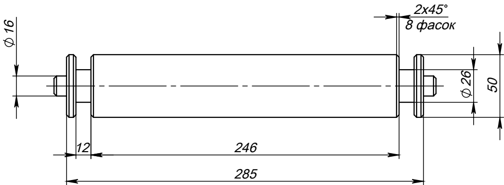
Поз.2 (Каток)
